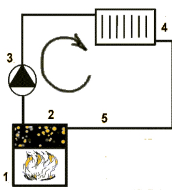
1.Котел 2. Подающая труба 3.Насос 4.Радиатор 5.Обратная труба
